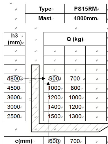
Fig. 9: Diagrama de sustentación residual
