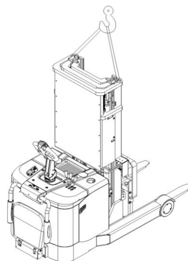
Figura 5: Levantamiento con grúa
